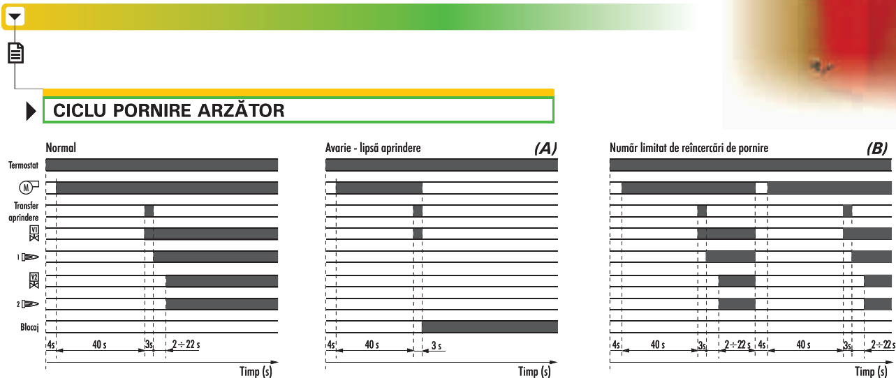
(A) Blocarea arzătorului este semnalizată de LED.
