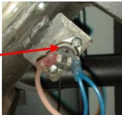
Senzor de detecție inversare a flăcării 105 grade C
