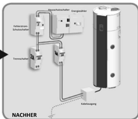
Installation der Warmwasser-Wärmepumpe
